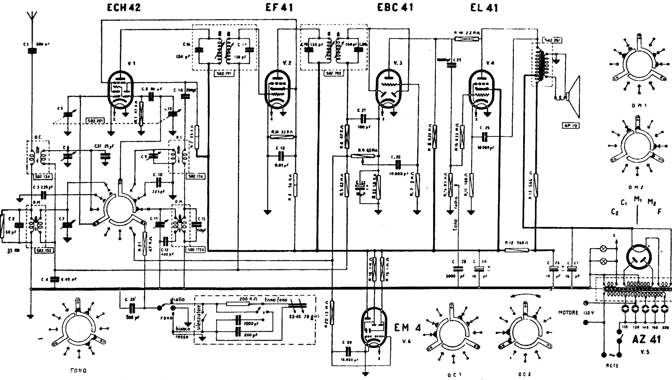
VOCE DEL PADRONE - Mod. Marconi 1543. Radiogrammfono da tavolo. Quattro gamme d'onda: OM1: 430-570; OM2: 187-440 m; OC1: 38,5-52 m; OC2: 18-38,5 m. Complesso giradischi a tre velocità, rivelatore con due puntine commutabili per dischi normali a 78 giri e microscolco a 33 e 45 giri. Potenza d'uscita 4 watt. Media frequenza 465 kc.
